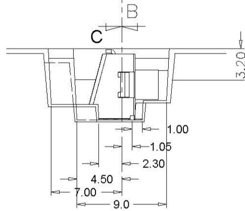
A-A Section
